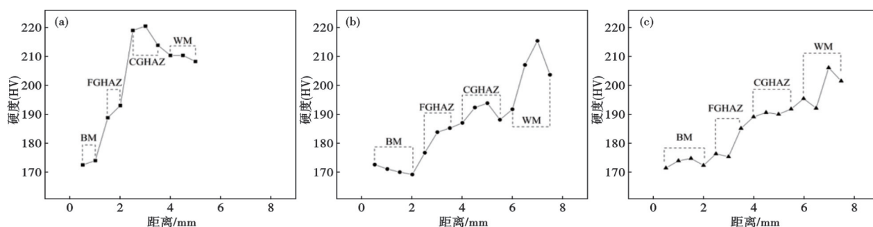
图6 FH420钢三种焊接接头的硬度分布:(a)二氧化碳气体保护焊,(b)单丝埋弧焊,(c)双丝埋弧焊
