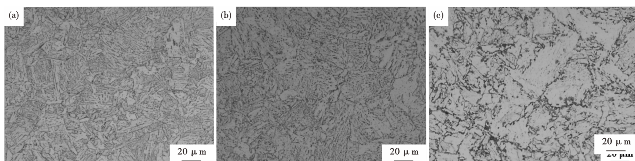
图4 FH420钢三种焊接接头粗晶热影响区的微观组织形貌:(a)二氧化碳气体保护焊,(b)单丝埋弧焊,(c)双丝埋弧焊
