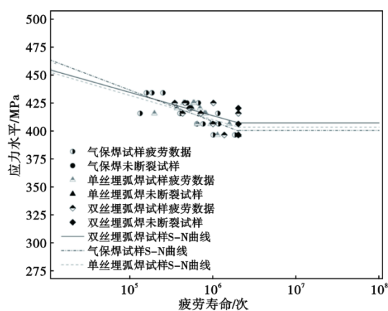
图7 FH420钢三种焊接接头的疲劳S-N曲线
