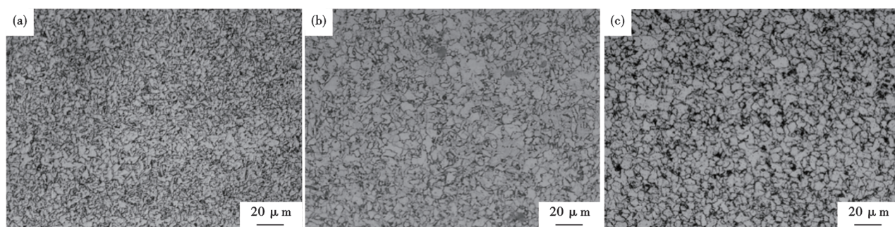
图3 FH420钢三种焊接接头细晶热影响区的微观组织形貌:(a)二氧化碳气体保护焊,(b)单丝埋弧焊,(c)双丝埋弧焊
