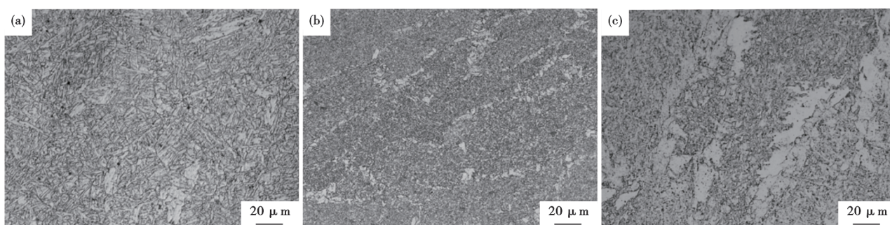
图5 FH420钢三种焊接接头焊缝的微观组织形貌:(a)二氧化碳气体保护焊,(b)单丝埋弧焊,(c)双丝埋弧焊
