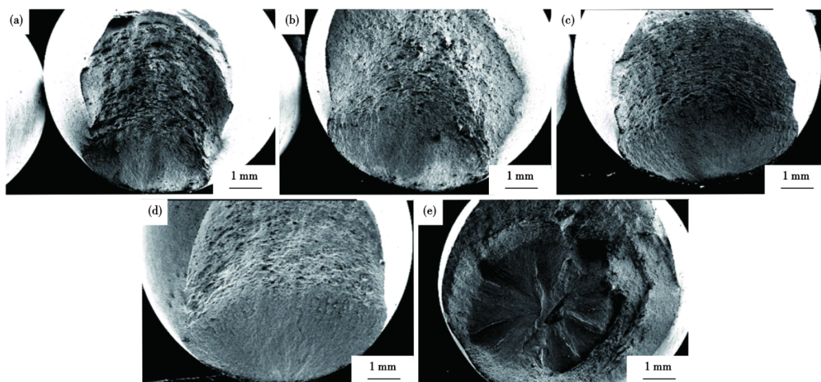
图 8 不同应力水平下 FH420 钢气保焊焊接接头宏观断口形貌: (a) 420 MPa, (b) 410 MPa, (c) 400 MPa, (d) 390 MPa, (e) 380 MPa Fig. 8 Macroscopic fracture morphology of FH420 steel gas shielded welding joint under different stress levels : (a) 420 MPa, (b) 410 MPa, (c) 400 MPa, (d) 390 MPa, (e) 380 MPa
