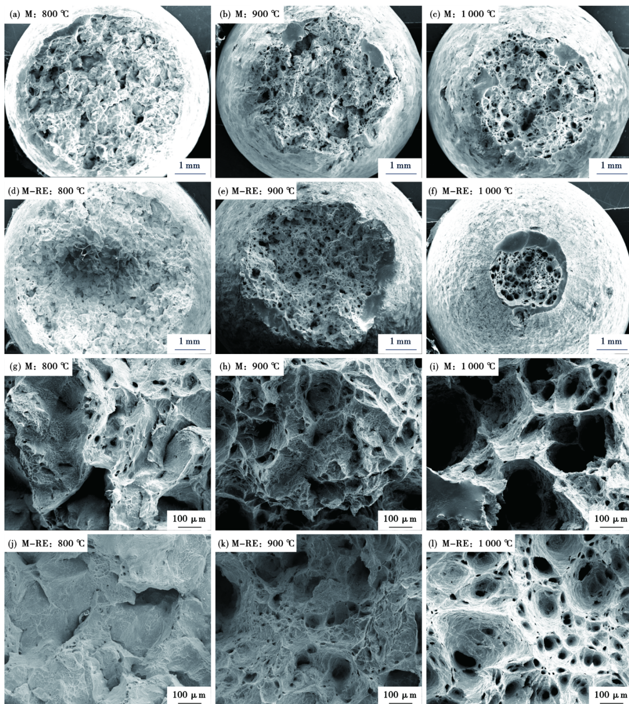
图9 800~1 100℃时高温拉伸断口放大图:(a)M,800℃;(b)M,900℃;(c)M,1 000℃;(d)M-RE,800℃;(e)M-RE,900℃;(f)M-RE,1 000℃;(g)M,800℃;(h)M,900℃;(i)M,1 000℃;(j)M-RE,800℃;(k)M-RE,800℃;(l)M-RE,800℃ Fig. 9 High temperature fracture morphology of medium manganese steel at 800 °C–1 200 °C: (a)M, 800 °C; (b)M, 900 °C; (c)M, 1 000 °C; (d)M-RE, 800 °C; (e)M-RE, 900 °C; (f)M-RE, 1 000 °C; (g)M, 800 °C; (h)M, 900 °C; (i)M, 1 000 °C; (j)M-RE, 800 °C; (k)M-RE, 800 °C; (l)M-RE, 800 °C
