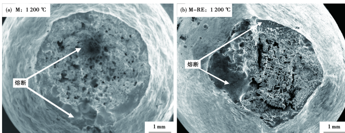
图7 中锰钢 1200 °C时的高温熔断断面:(a)M钢,(b)M-RE钢
