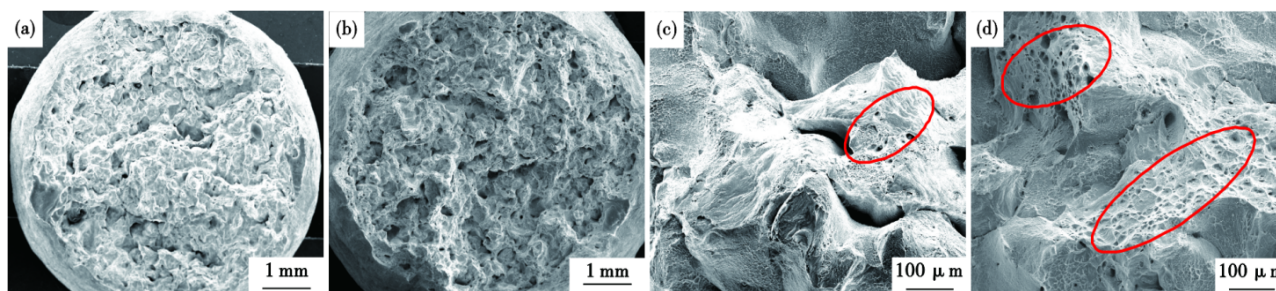
图8 中锰钢 700 °C时的高温断面形貌:(a)M;(b)M-RE;(c)M;(d)M-RE
