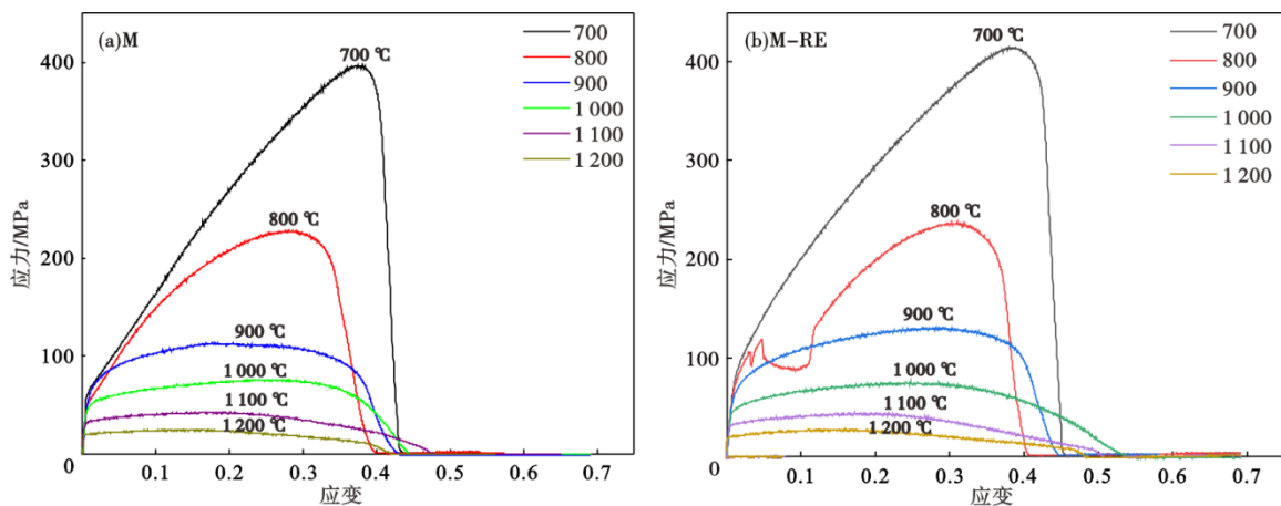
图3 中锰钢真应力应变曲线:(a)M钢,(b)M-RE钢
