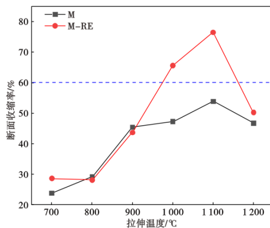
图6 中锰钢不同温度下断面收缩率
