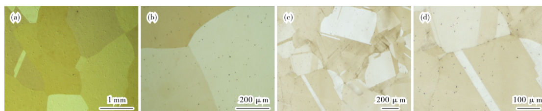
图 1 Fe-1.4C-8Mn-2Al 钢中奥氏体晶粒形貌:(a) (b) 铸造+固溶态, (c) (d) 热轧+固溶态
