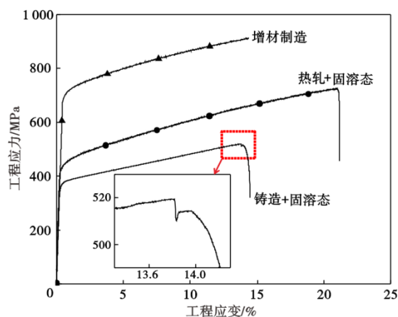
图3 Fe-1.4C-8Mn-2Al 实验钢拉伸应力-应变曲线
