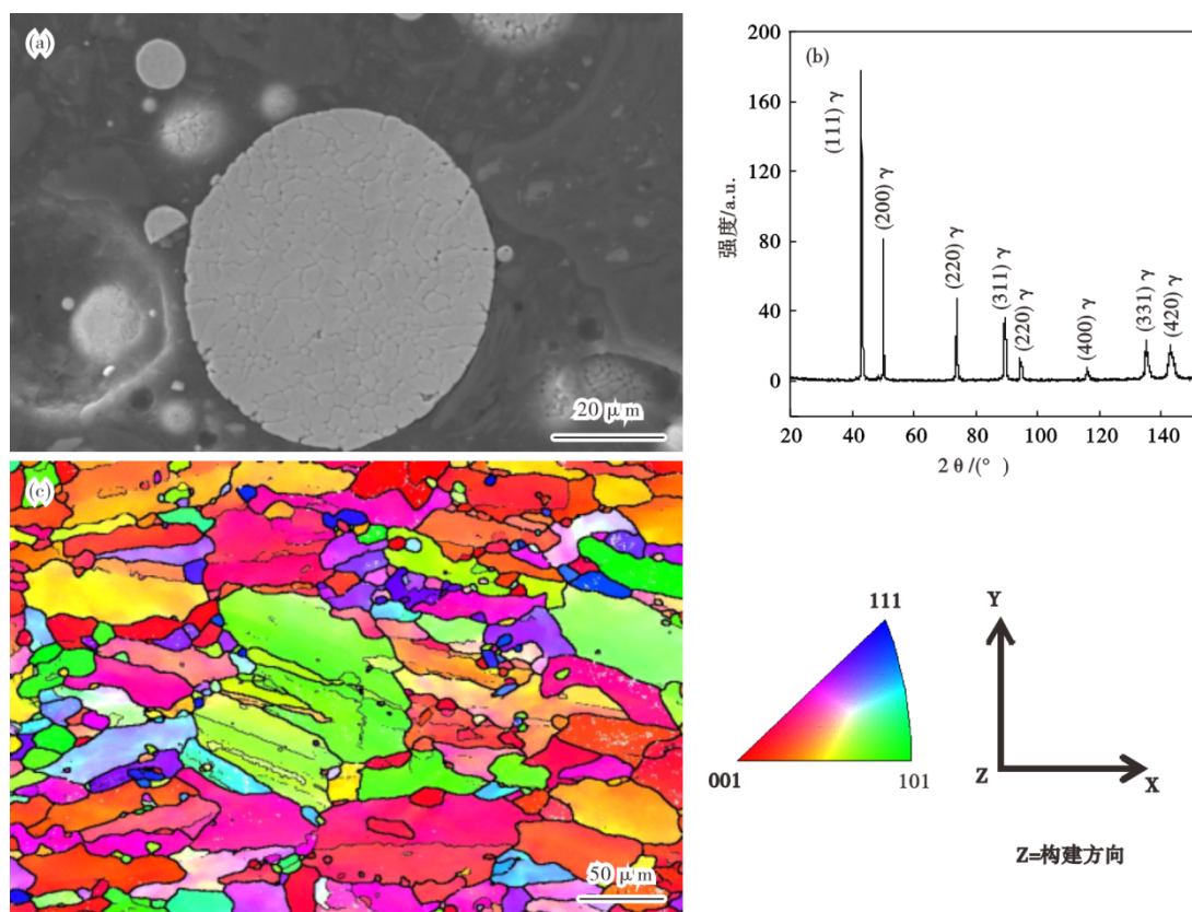
图2 增材制造 Fe-1.4C-8Mn-2Al 实验钢组织分析: (a) 粉末形貌, (b) 粉末 XRD 图谱, (c) EBSD-IPF 图
