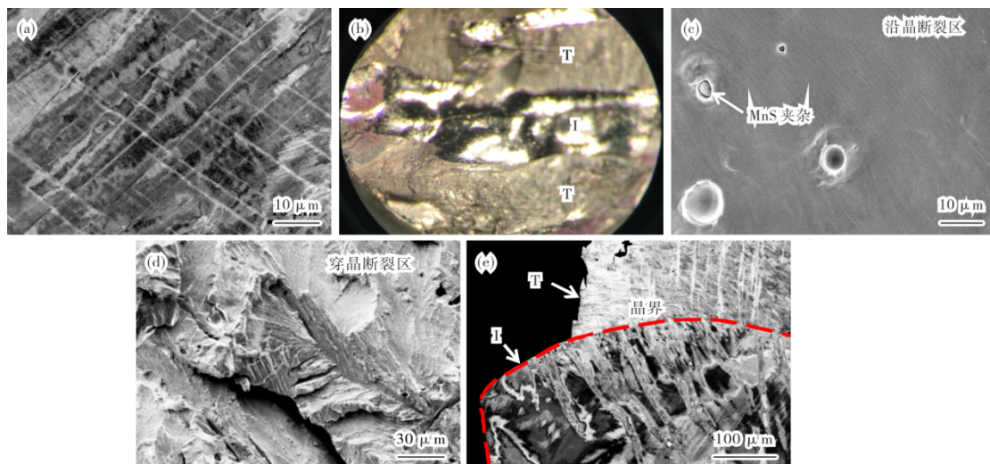
图4 铸造+固溶态Fe-1.4C-8Mn-2Al实验钢组织:(a) ECCI组织图,(b) 断口形貌,(c) 沿晶断裂区断口形貌,(d) 穿晶断裂区断口形貌,(e) 穿晶断裂区和沿晶断裂区交界处ECCI组织(拉伸方向为水平方向)
