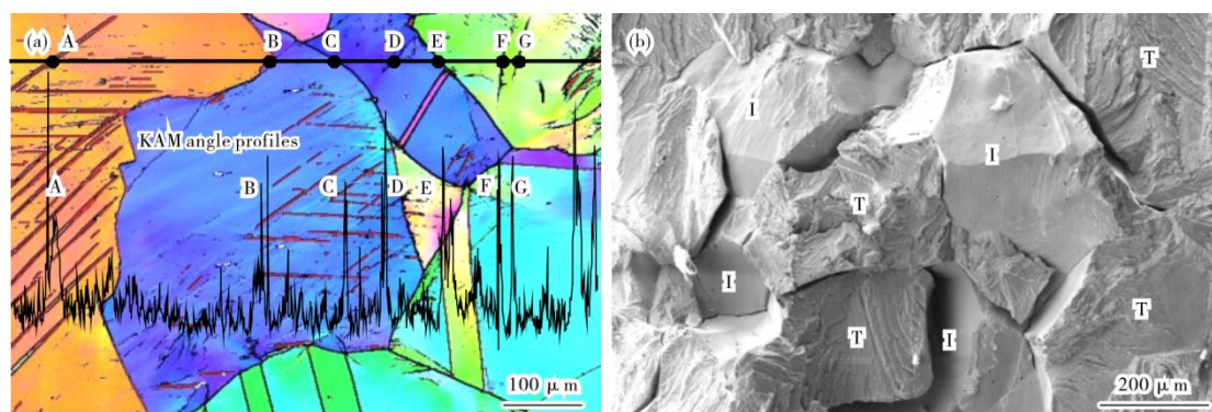
图5 热轧+固溶态 Fe-1.4C-8Mn-2Al 实验钢组织: (a) EBSD-IPF 组织图, (b) 断口形貌
