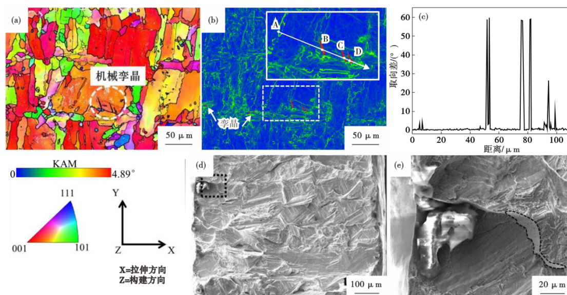
图6 增材制造 Fe-1.4C-8Mn-2Al 实验钢组织: (a) EBSD-IPF 组织图, (b) KAM 图, (c) 取向差分布曲线, (d) 断口形貌, (e) 图d中方框组织放大图
